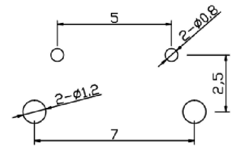
PCB. 焊接图
