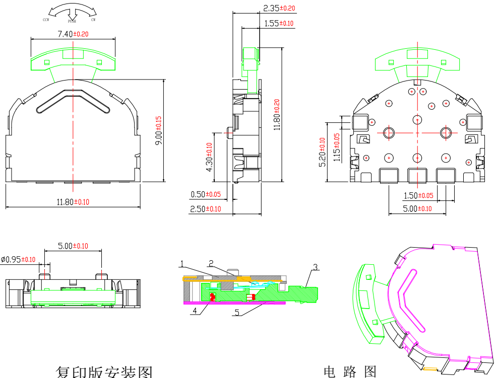
复印版安装图
