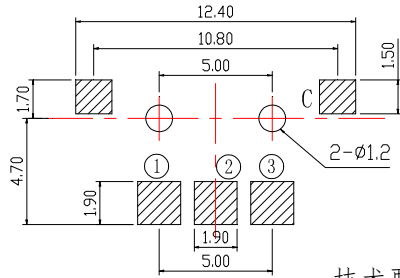
复印版安装图
